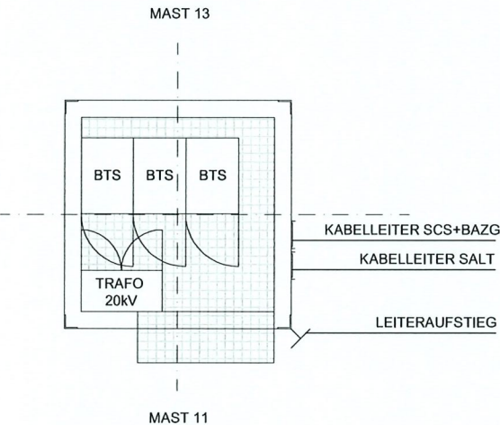
SCHNITT D-D 1:100
