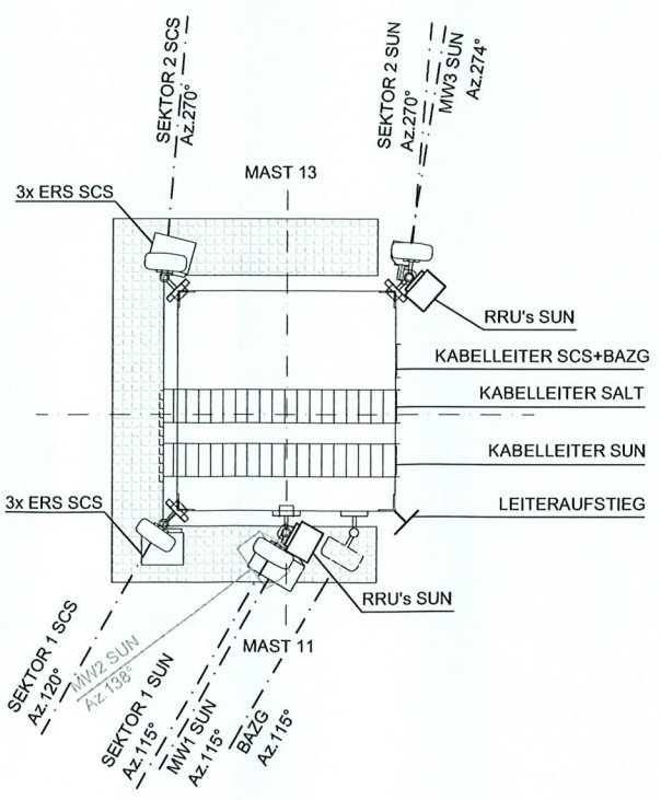
SCHNITT B-B 1:100
