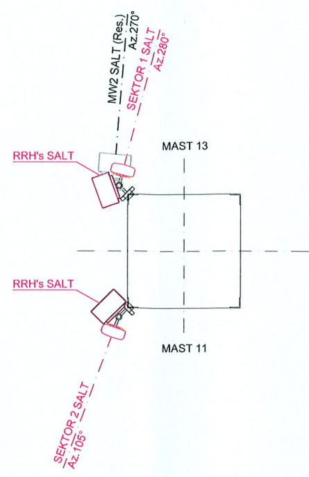
SCHNITT A-A 1:100
